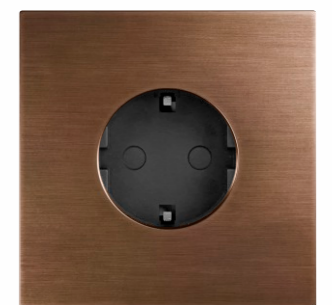
Рамка на 1 пост, «Берлин Премиум», латунь, сатин патинир. античная, Модуль розетки Schuko, «Берлин Премиум», Чёрный
